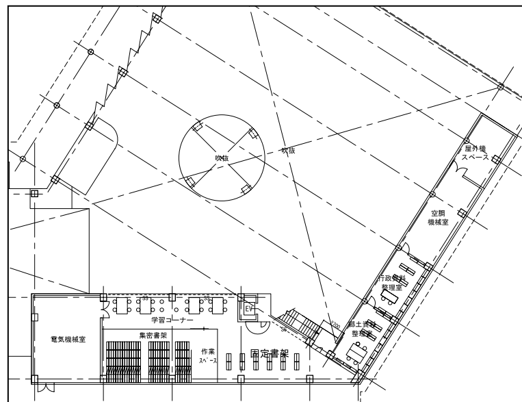
●図書館1階平面図
