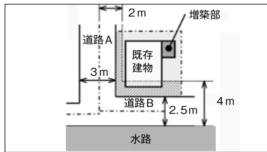
セットバックについての事例（2）
