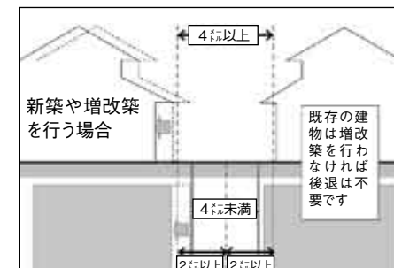
接道義務・敷地後退
