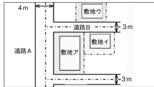
セットバックについての事例（1）
